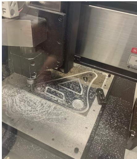
図1 ベルクランク製作の様子
